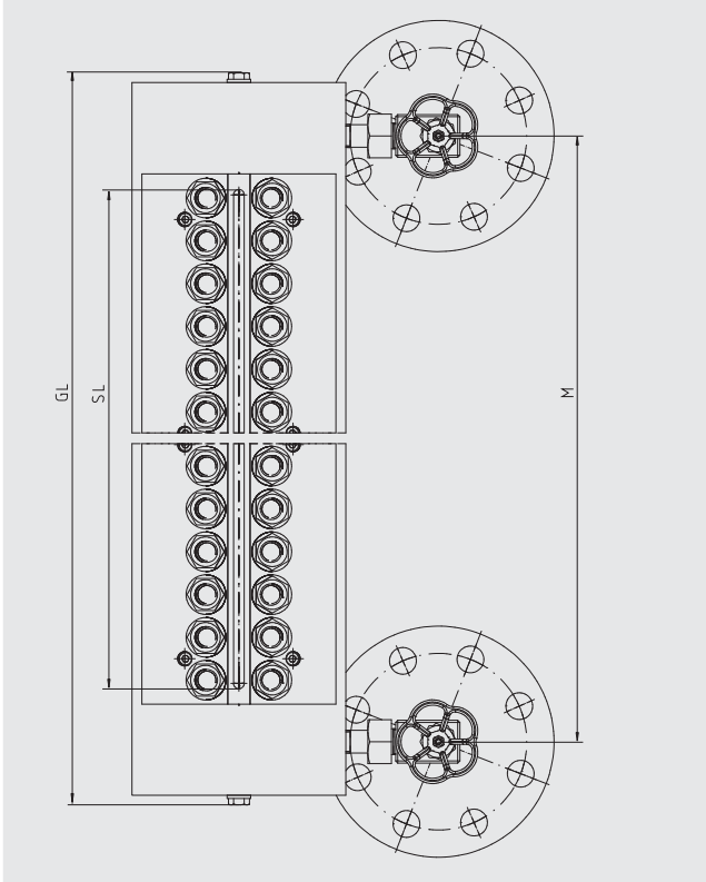
Ausführung mit Ventilkopf, seitlich, Typ LGV-52
