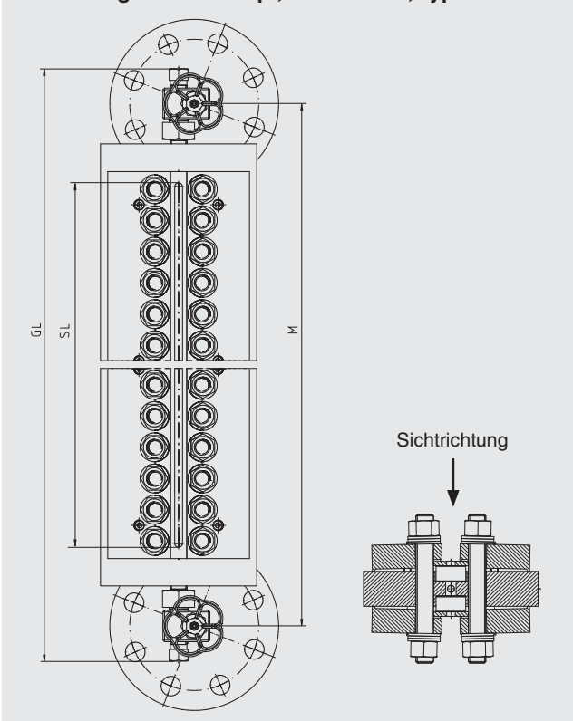
Ausführung mit Ventilkopf, oben/unten, Typ LGV-53
