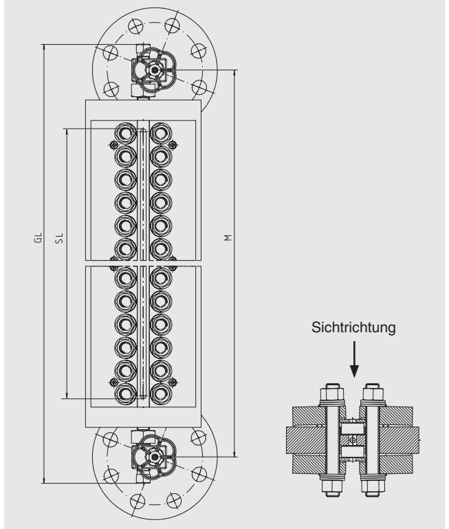
Ausführung mit Ventilkopf, oben/unten, Typ LGV-53
